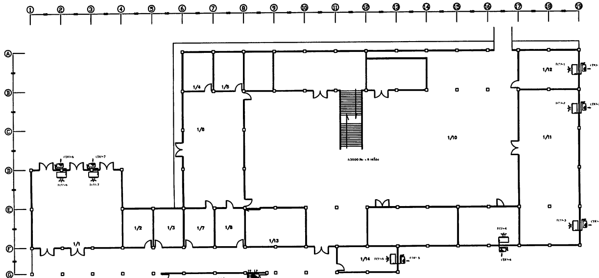
แปลนติดตั้งเครื่องปรับอากาศห้องสมุด ชั้น 1
